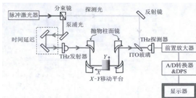
图3 太赫兹扫描成像系统原理图
