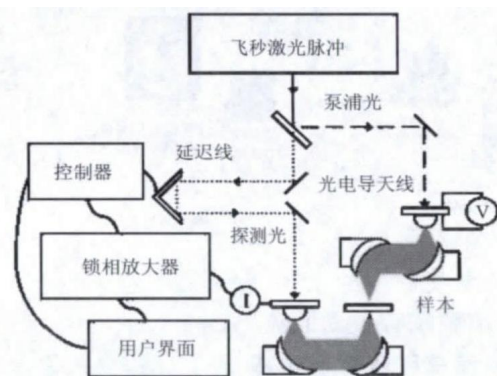
图2 使用光电导天线的典型THz-TDS透射系统原理图
