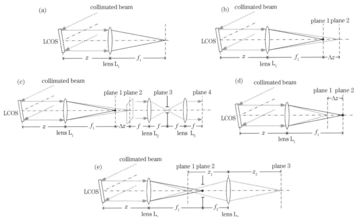
图2 光学示意图。(a)原先的全息显示系统;(b)发散球面波相位;(c)发散球面波相位+4f系统;(d)会聚球面波相位;(e)提出的全息显示系统
