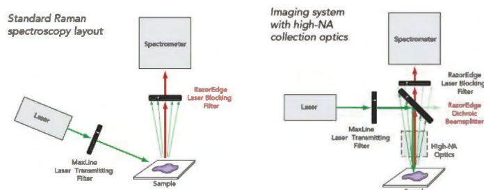
常规拉曼系统图
