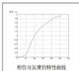
RSLM-HD70-NIR2 相位与灰度的特性曲线
